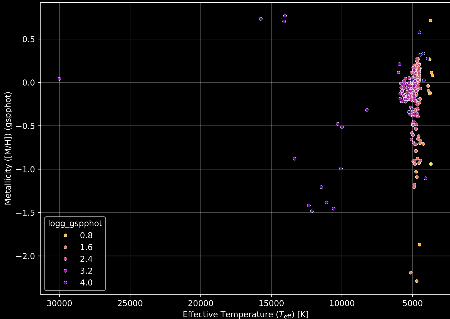
APOGEE DR17 Field: [214-08] Stellar Population Parameters (n= 308)
